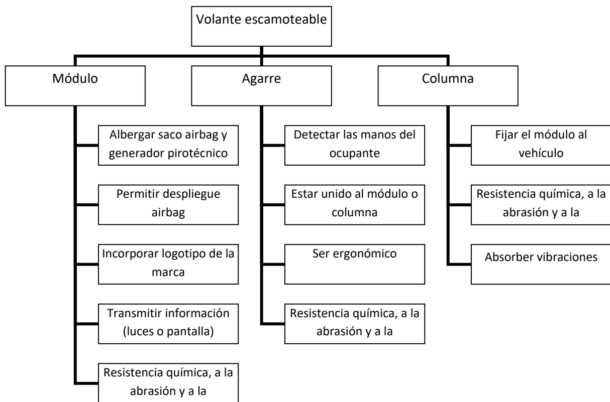
Fig. 3. Diagrama de funciones de cada subsistema.
