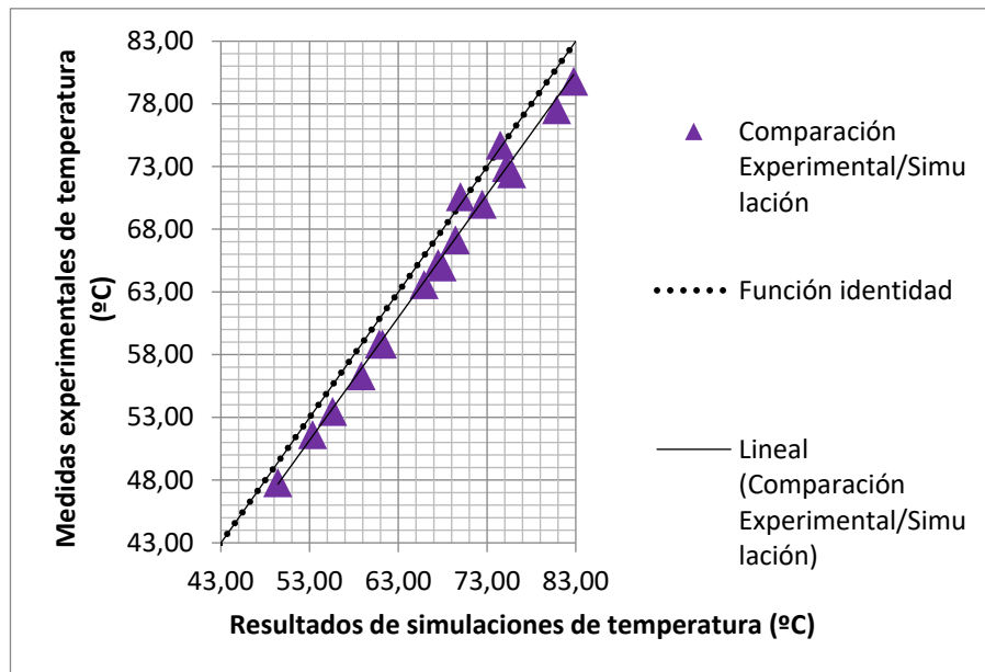
Fig. 4. Comparación entre resultados experimentales y simulados.
