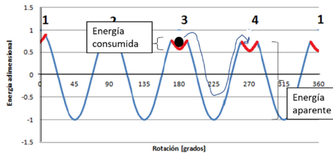
Fig. 2. Energía potencial almacenada.
