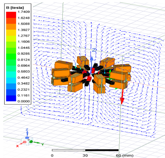
Fig. 6. Vectores de densidad de campo magnético en el plano YZ del dispositivo.
