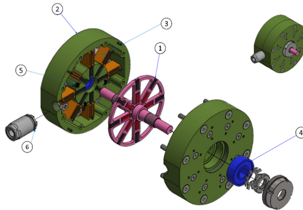
Fig. 3. Diseño detallado del actuador VALMAC.
