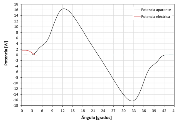
Fig. 14. Potencia vs. posición del rotor.
