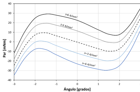
Fig. 10. Influencia de la corriente en las bobinas en función de la posición del rotor.
