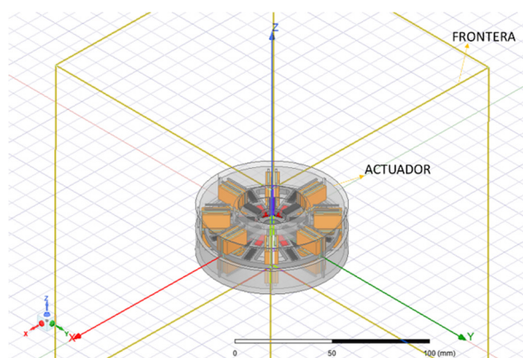
Fig. 5. Modelo magnetoestático de elementos finitos.
