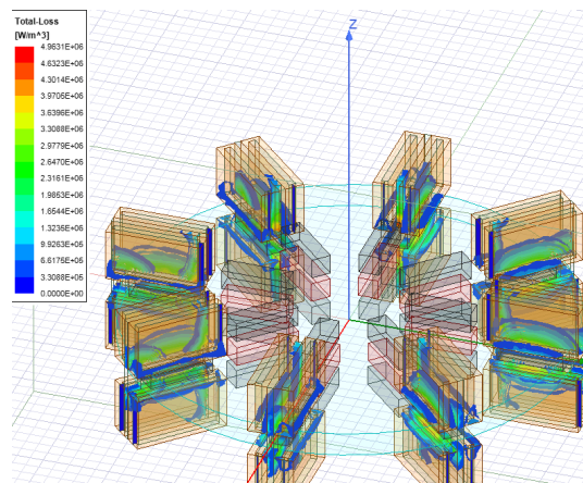
Fig. 7. Pérdidas magnéticas específicas durante un instante de la simulación.
