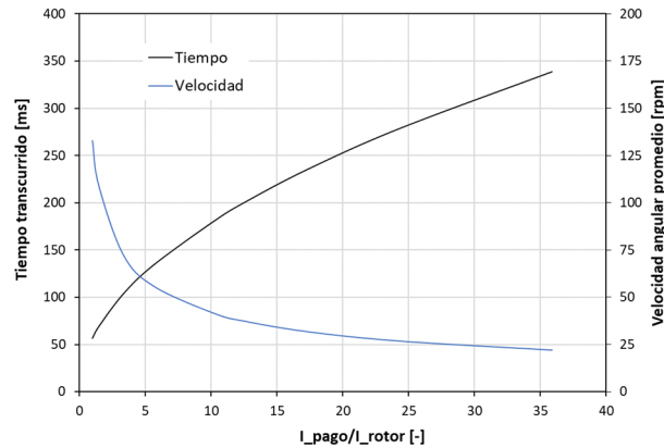
Fig. 13. Velocidad promedio y tiempo de cambio de posición vs. relación de momentos de inercia.
