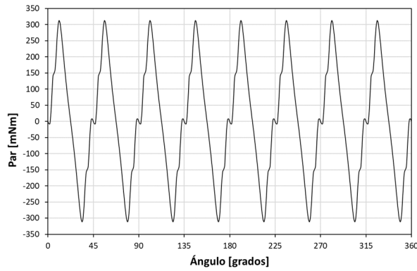
Fig. 8. Par vs. Ángulo de giro del rotor.
