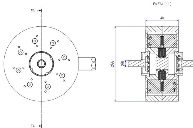
Fig. 4. Vista en sección y dimensiones generales.
