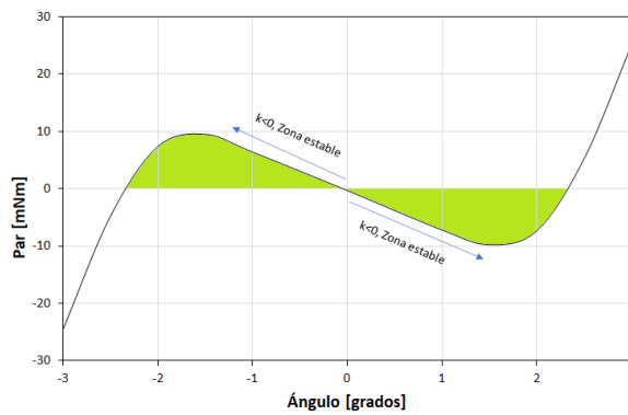
Fig. 9. Posición de equilibrio estable.
