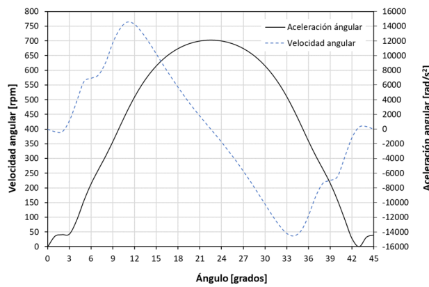
Fig. 11. Velocidad y aceleración angular vs. ángulo de giro del rotor.
