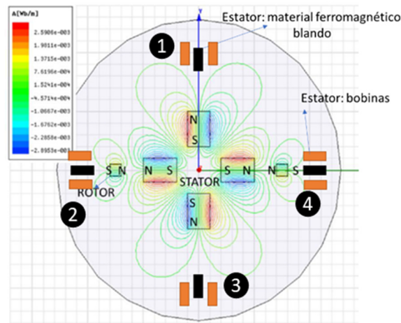
Fig. 1. Vista en planta y principio de funcionamiento.
