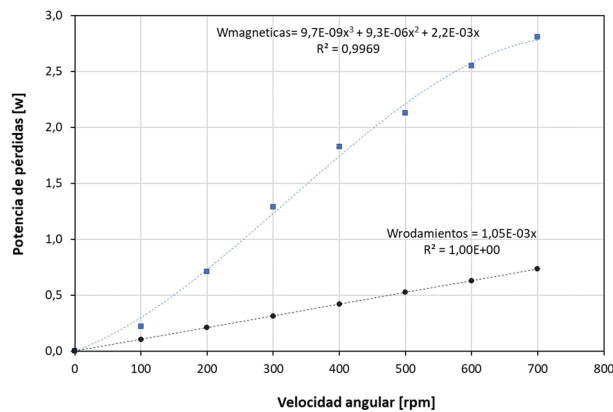
Fig. 15. Pérdidas vs. velocidad angular del rotor.
