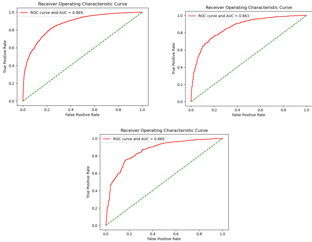
Fig. 3. Curvas ROC para clasificación binaria, a) para entrenamiento, b) validación, y c) test.
