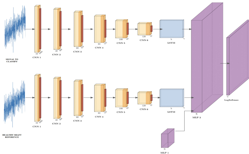
Fig. 2. Arquitectura de la red neuronal utilizada.
