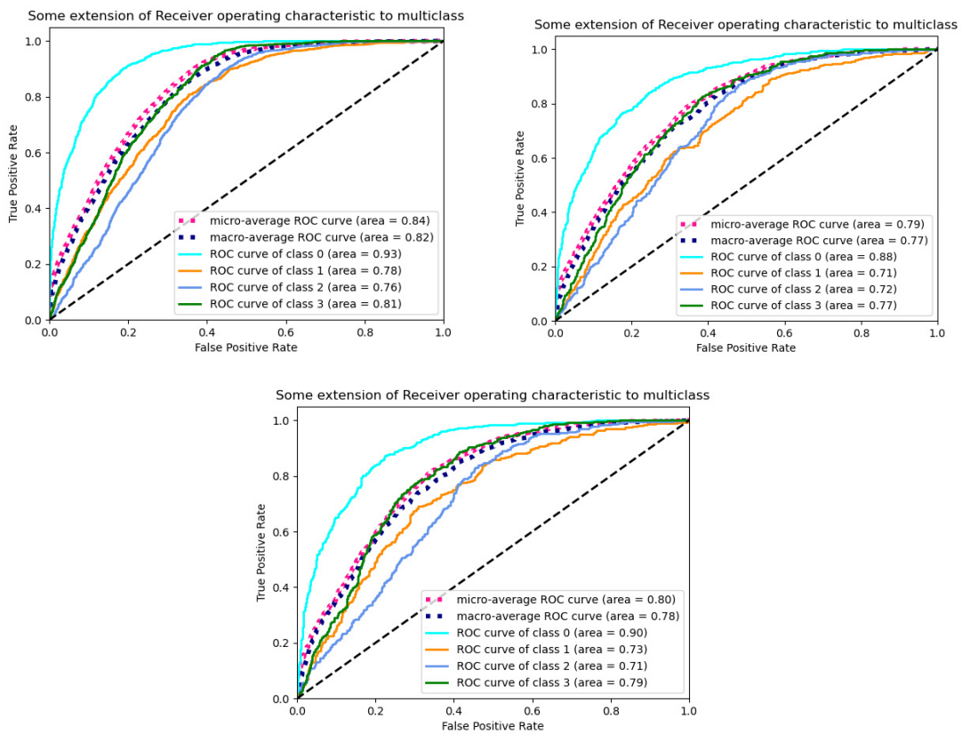
Fig. 4. Curvas ROC para clasificación multiclase, a) para entrenamiento, b) validación, y c) test.
