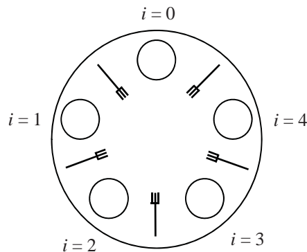
Figura 16 – Ubicación de los filósofos en la mesa
